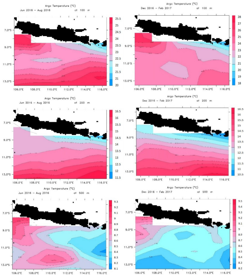
Gambar 8a. Subsurface temperature di kedalaman 100 m , 200 m dan 500 m pada musim timur.
