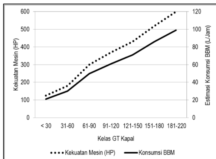
Gambar 5. Estimasi konsumsi BBM kapal pukat cincin pelagis besar yang berbasis di Bitung. Figure 5. Estimation of fuel consumption of the purse seiners based at Bitung.
