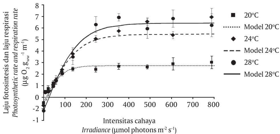
Gambar 8. Model kurva P-I Kappaphycus sp. (strain Sumba) pada suhu 20°C, 24°C, dan 28°C yang diperoleh dengan cara memplotkan pada kurva P-I dengan menggunakan rumus P = \{P_{\max} \times \tanh(\alpha / P_{\max} \times I)\} + R_d
