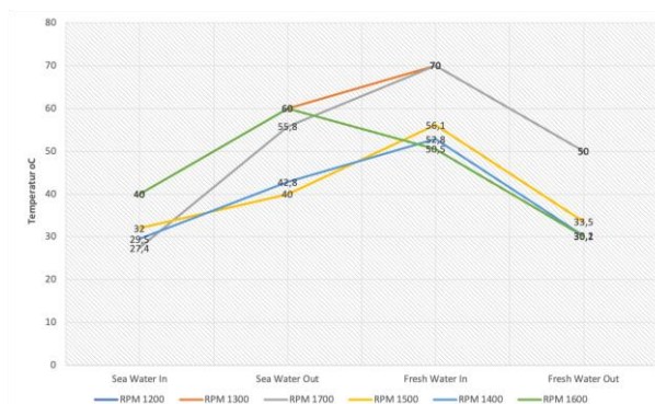
Gambar 2. Perbandingan RPM Mesin Induk Terhadap Temperatur Air Pendingin
