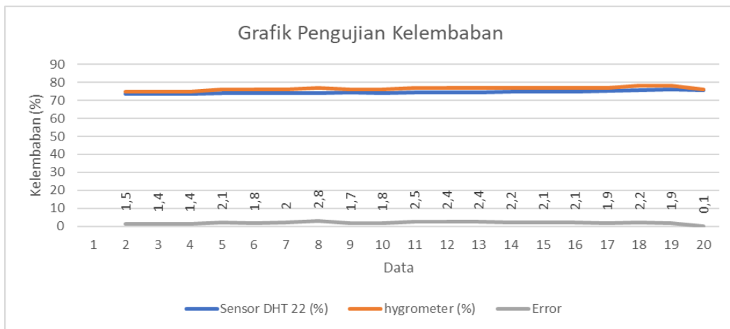
Gambar 11. grafik Pengujian Kelembaban
