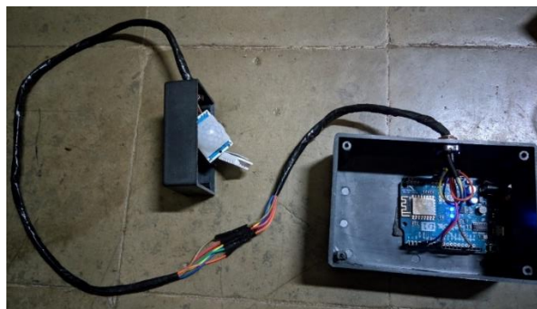
Gambar 7. Tampilan Alat
