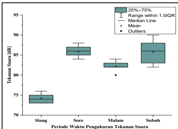
Gambar 3. Rata-rata tekanan suara (dB) pada Siang hari, Sore hari, Malam hari, dan dini hari
